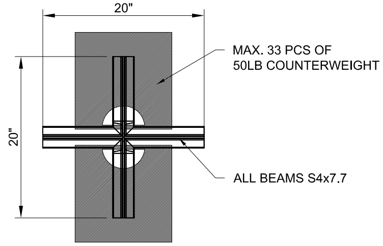
1 PLAN VIEW SCALE: 1" = 1'-0"
